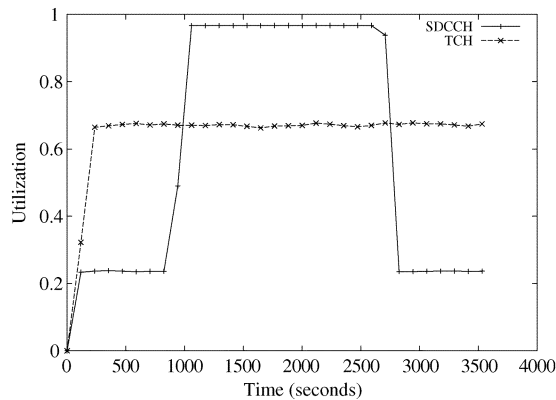
Fig. 20. Channel utilization under DCA.
